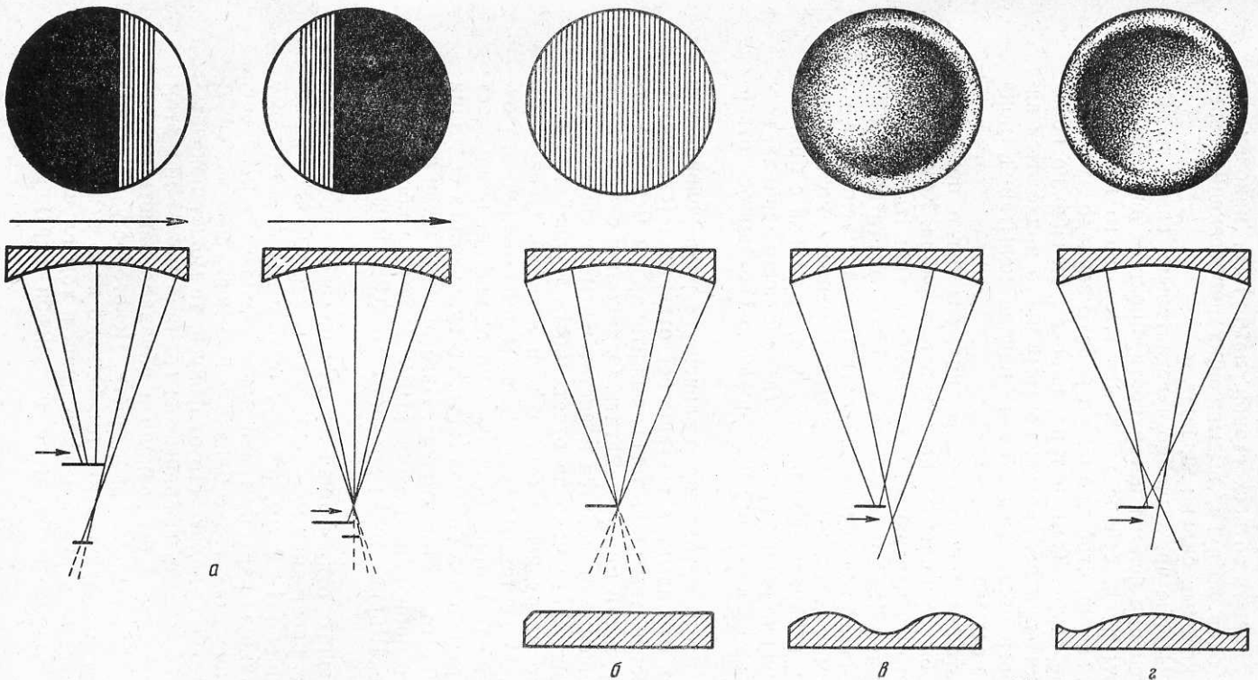
Рис. 3. Вид теней Фуко, даваемых поверхностями различного рода
