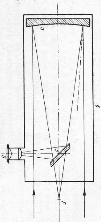
Рис. 1. Схема рефлектора системы Ньютона a — главное вогнутое зеркало, образующее изображение светила в F (главный фокус); b — маленькое плоское зеркальце, поставленное перед фокусом под углом в 45^\circ к оптической оси, отражает конус лучей в боковое отверстие трубы, где его рассматривают в окуляр o ; v — труба
