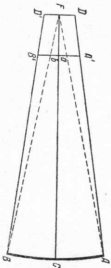
Рис. 4. Определение размеров плоского малого зеркальца для рефлектора системы Ньютона AB — главное вогнутое зеркало; главный фокус его в точке F на оптической оси CF , DD' — поле зрения в фокальной плоскости. Малая ось плоского зеркальца должна быть равна A'B' , а не ab , так как поле зрения не точка F , а кружок с поперечником DD'
