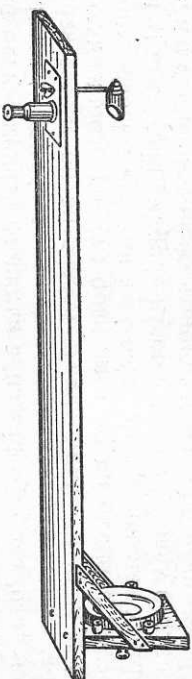
Рис. 6. «Чингисская доска» для предварительной монтировки. Описанное в тексте устройство окулярной части доски не сколько упрощено по сравнению с показанным на рисунке
