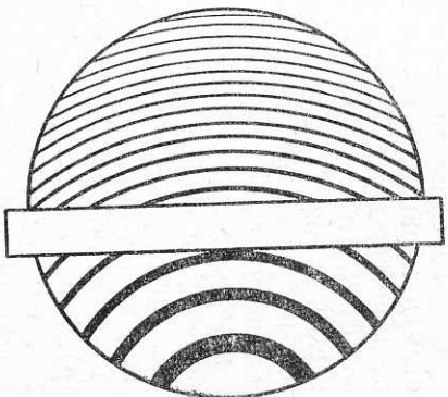
Рис. 5. Вид интерференционных полос в случае выпуклости испытываемого стекла (предполагается, что на него наложено в точности плоское пробное стекло). С правой стороны полосы шире и сильнее искривлены, что указывает на более тесное соприкосновение стекол. Приложенная линейка позволяет определить кривизну стекла (в данном случае выпуклость составляет около трех полос)
